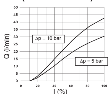
XDP.3.*.01.N (40 l/min P → A/B)
