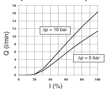
XDP.3.*.01.N (15 l/min P → A/B)
